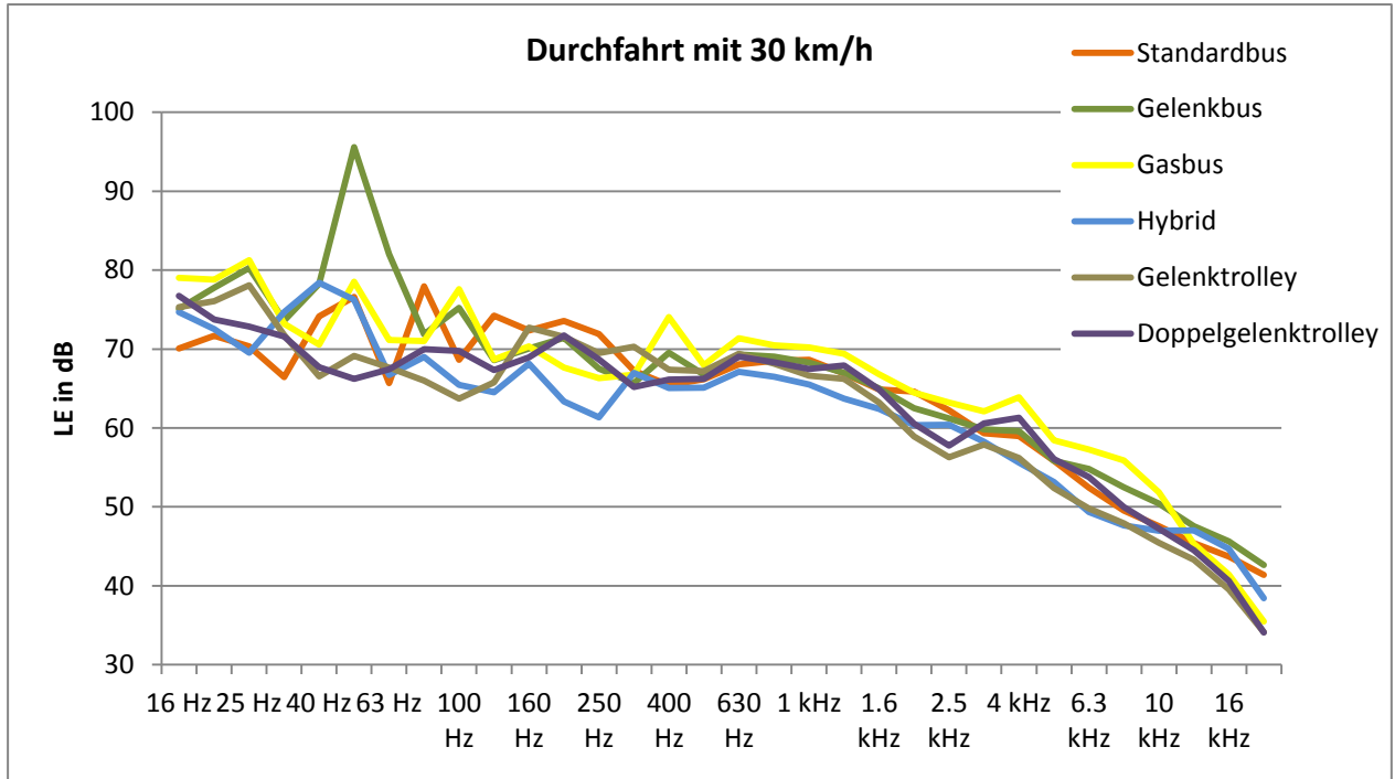
Abb. 4: Frequenzspektren der verschiedenen Kategorien bei einer Durchfahrt mit 30 km/h (ohne Belagsberücksichtigung)
