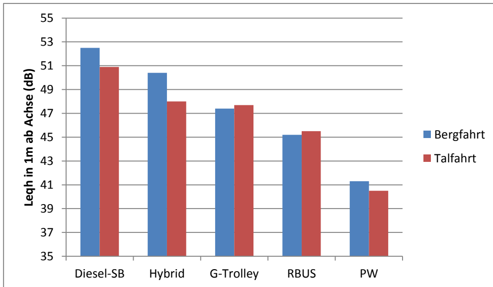
Abb. 22: Pegelunterschiede Berg- und Talfahrt der in Luzern gemessenen Busse
