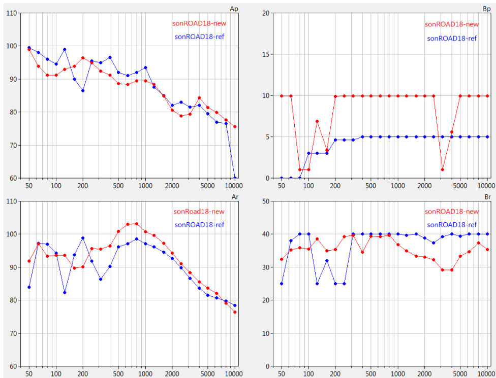
Abbildung 60: Spektrale Modellparameter in rot im Vergleich zu den Standardwerten SWISS10 cat 1 (blau).
