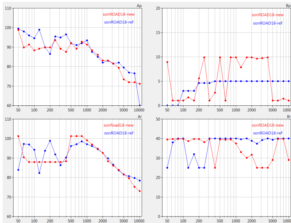
Abbildung 43: Spektrale Modellparameter in rot im Vergleich zu den Standardwerten SWISS10 cat 1 (blau).
