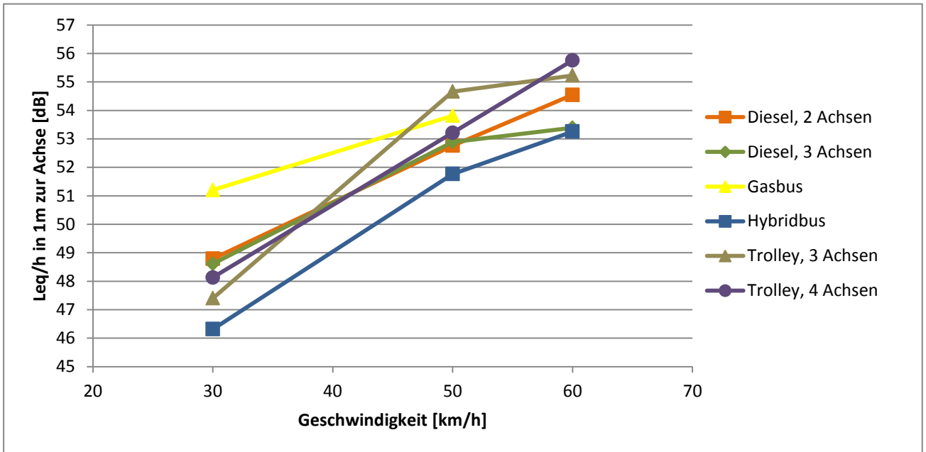
Abb. 21: Schalldruckpegel in Abhängigkeit der Geschwindigkeit pro Kategorie
