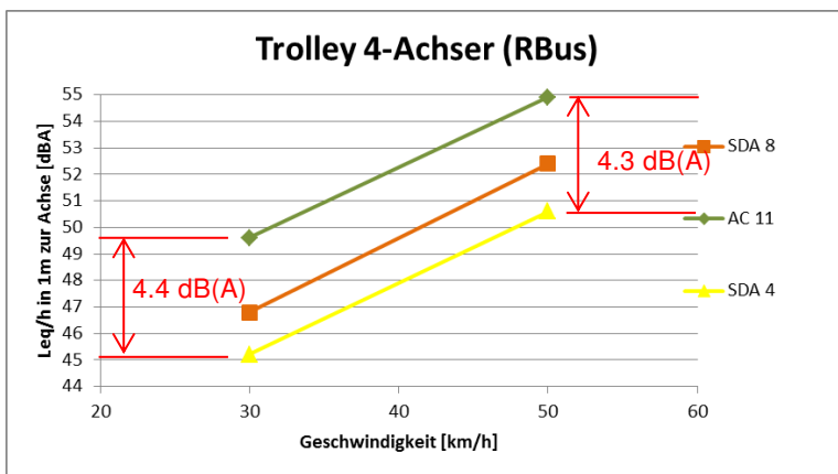
Abb. 13: Quellenwert (L q ) Trolley 4-Achser
