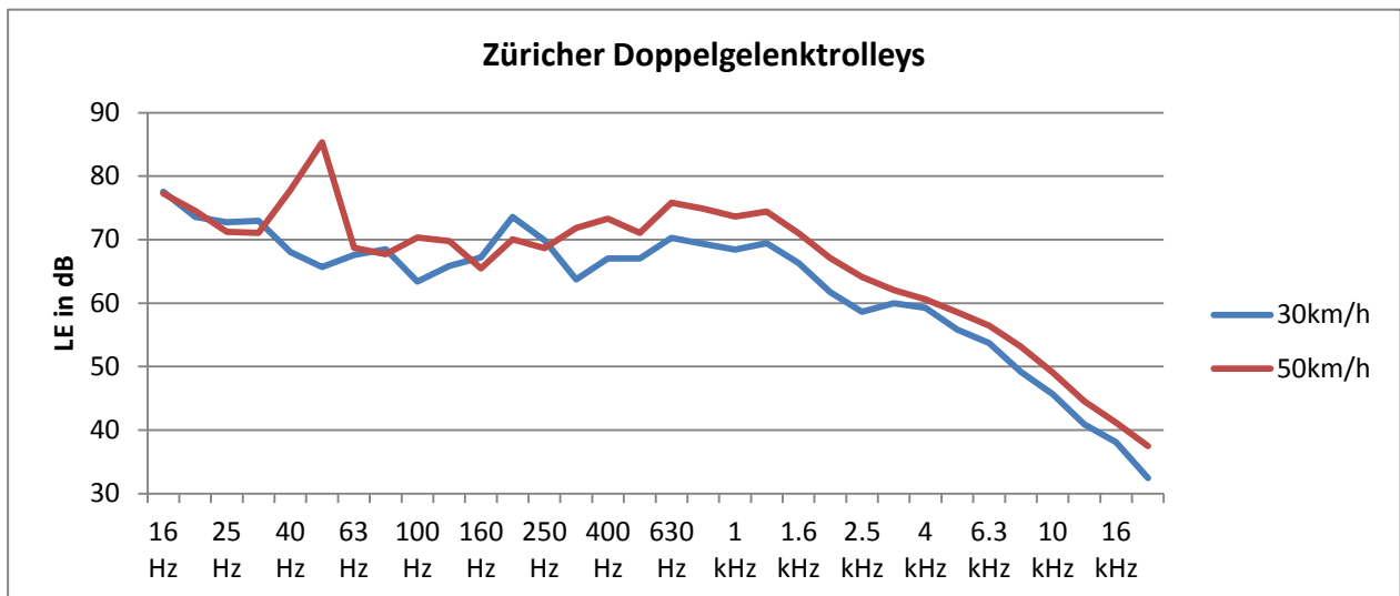
Abb. 9: Frequenzspektrum der Züricher Doppelgelenktrolleys
