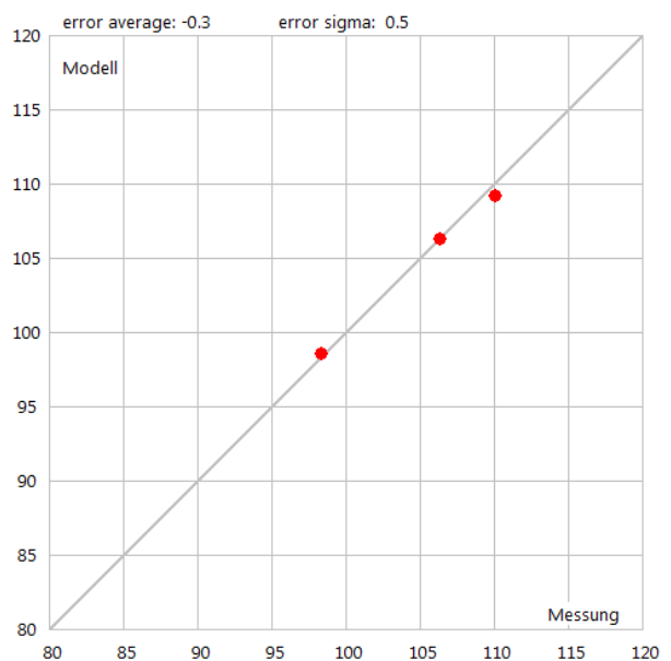
Abbildung 30: X-Y Plot der gemessenen und modellierten A-Summenpegel.
