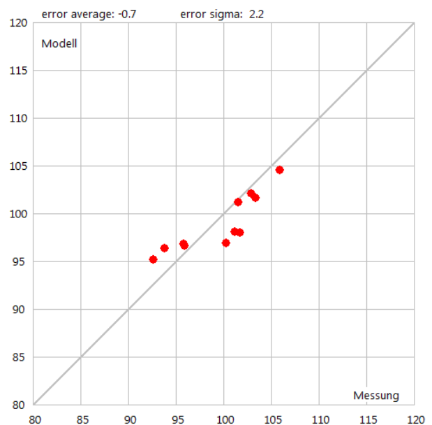
Abbildung 57: X-Y Plot der gemessenen und modellierten A-Summenpegel.
