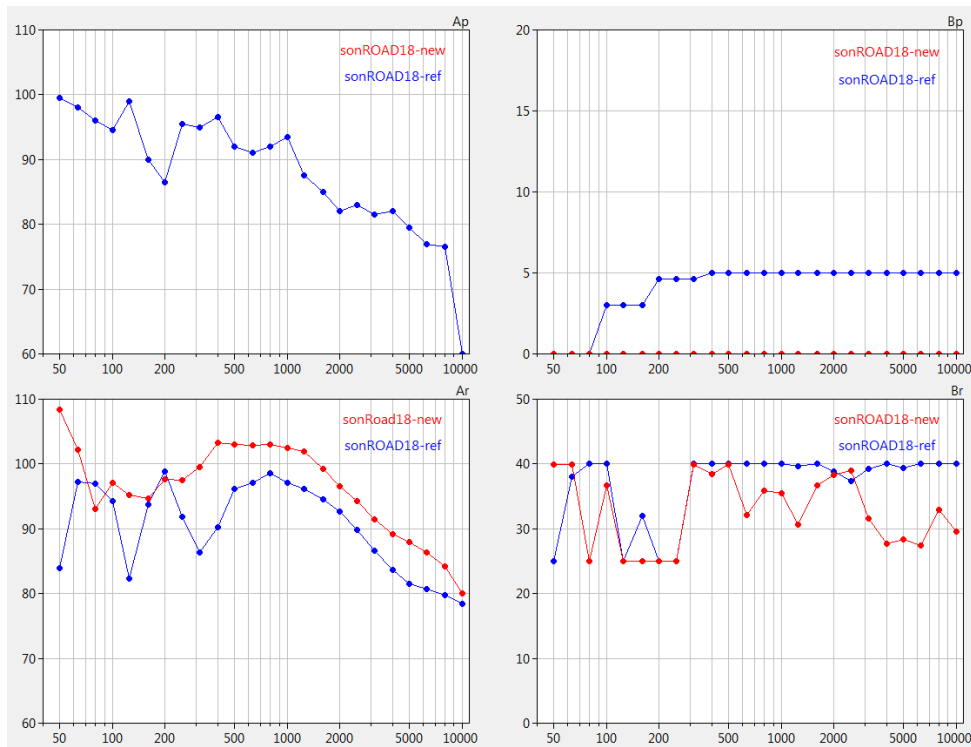
Abbildung 23: Spektrale Modellparameter in rot im Vergleich zu den Standardwerten SWISS10 cat 1 (blau).
