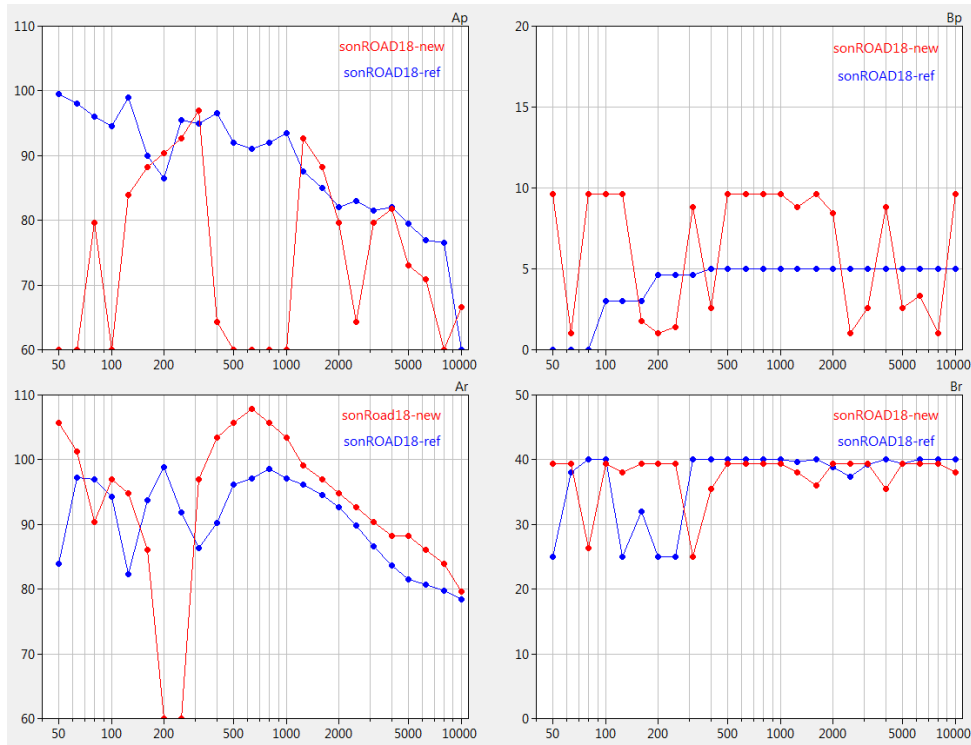
Abbildung 29: Spektrale Modellparameter in rot im Vergleich zu den Standardwerten SWISS10 cat 1 (blau).
