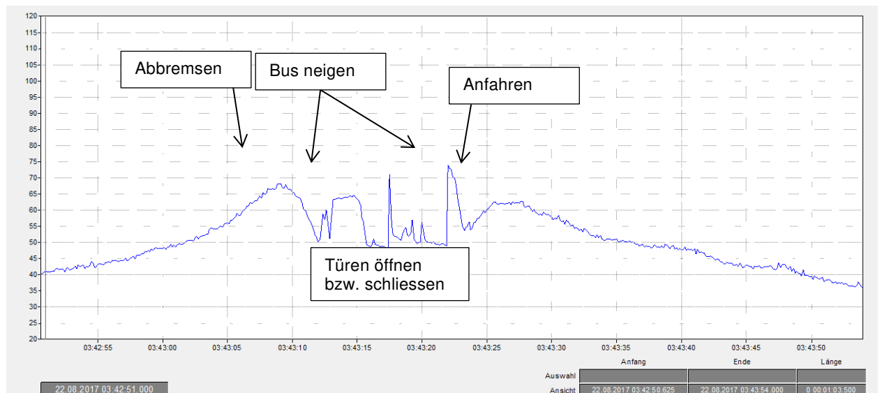
Abb. 23: Haltevorgang des Zürcher Bus Nr. 2.1, Doppelgelenktrolley, Kategorie Trolley
