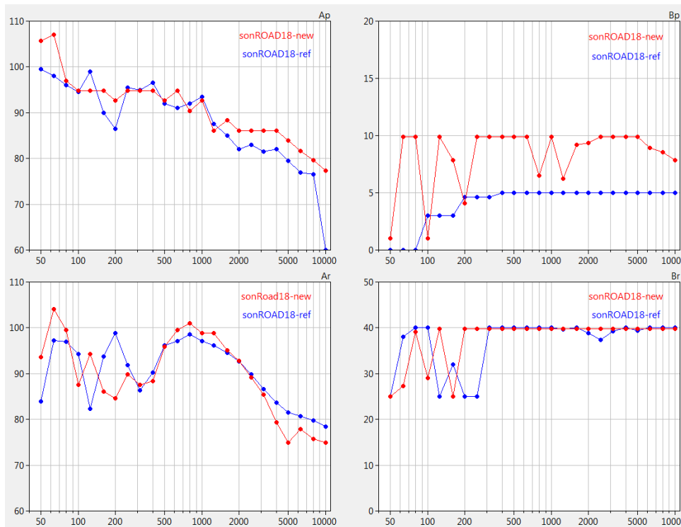
Abbildung 39: Spektrale Modellparameter in rot im Vergleich zu den Standardwerten SWISS10 cat 1 (blau).
