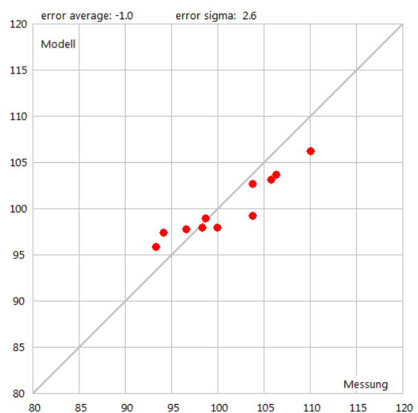
Abbildung 59: X-Y Plot der gemessenen und modellierten A-Summenpegel.
