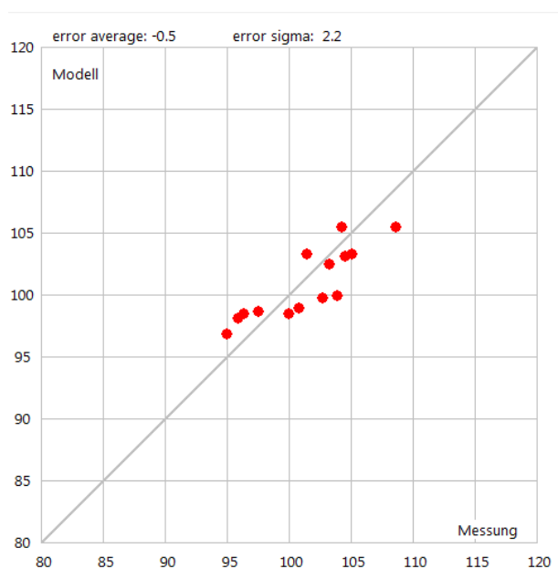
Abbildung 42: X-Y Plot der gemessenen und modellierten A-Summenpegel.
