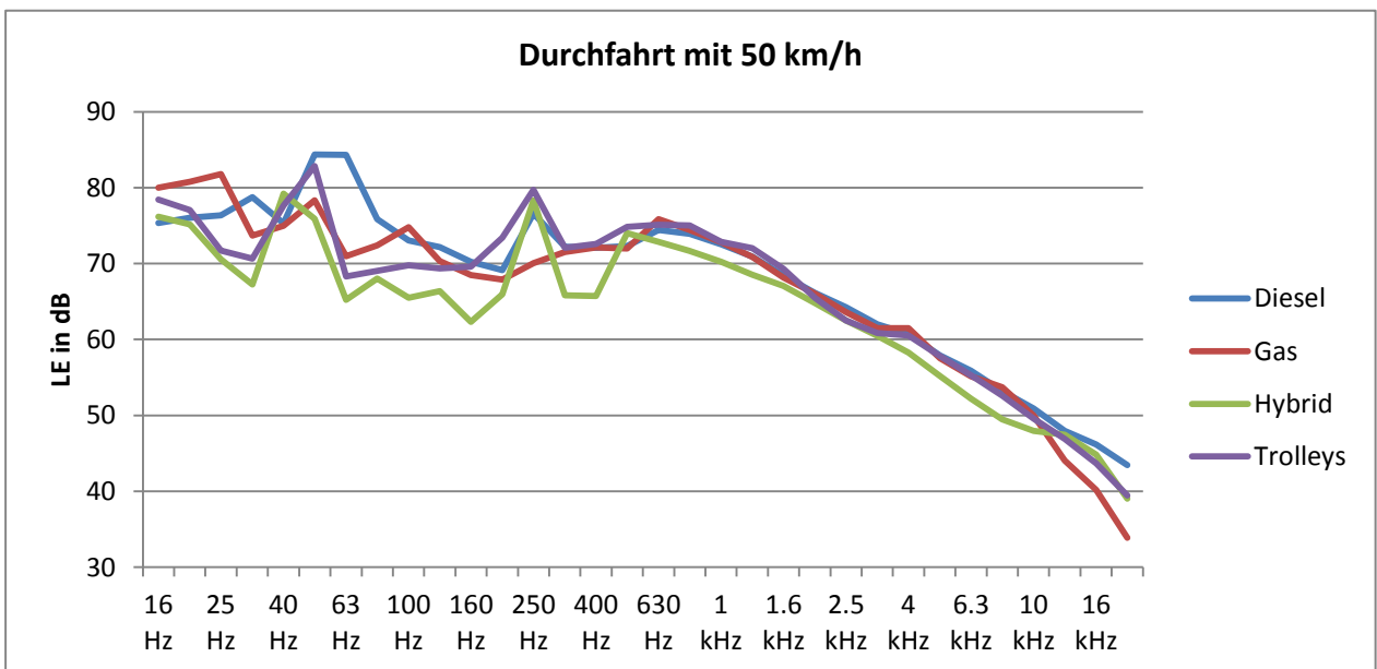
Abb. 7: Frequenzspektrum nach Antriebsart bei 50 km/h (ohne Belagsberücksichtigung)
