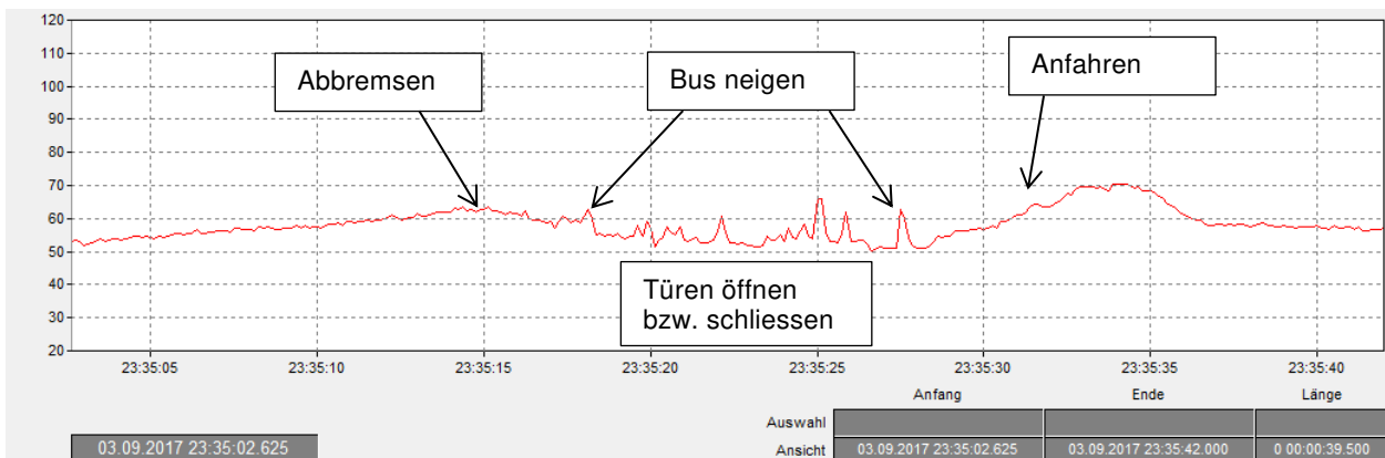
Abb. 26: Haltevorgang des Luzerner Bus Nr. 2, Hybridbus
