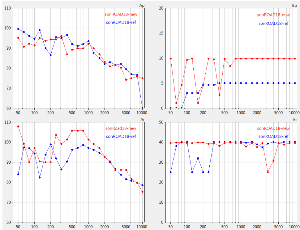
Abbildung 45: Spektrale Modellparameter in rot im Vergleich zu den Standardwerten SWISS10 cat 1 (blau).
