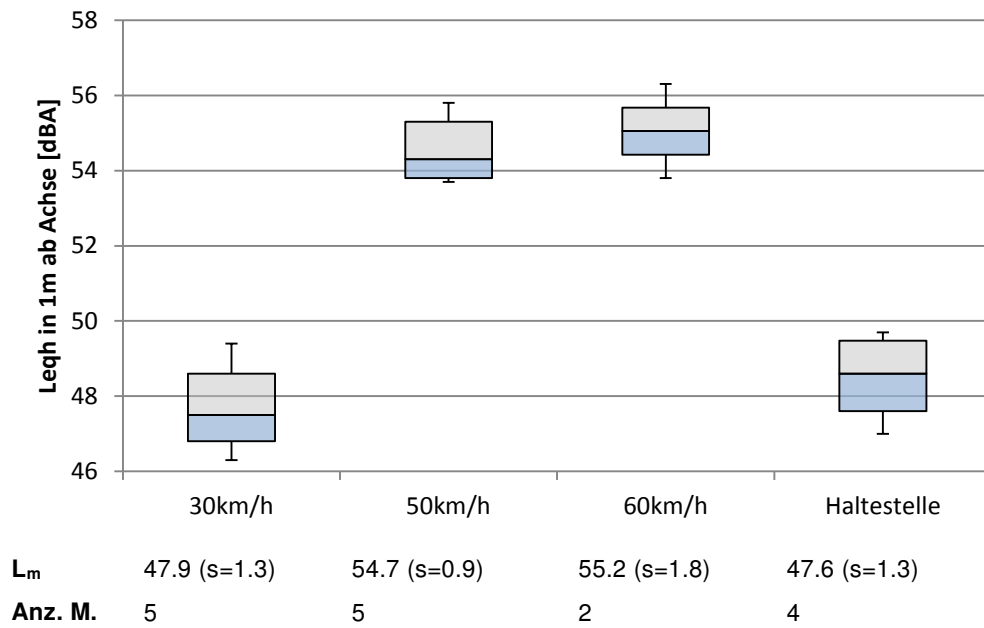
Abb. 19: Boxplots Kategorie Trolley, 3-Achser, Gelenktrolleybus
