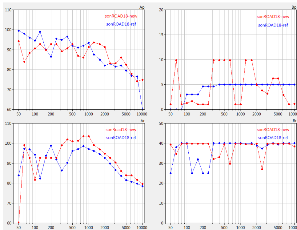
Abbildung 17: Spektrale Modellparameter in rot im Vergleich zu den Standardwerten SWISS10 cat 1 (blau).
