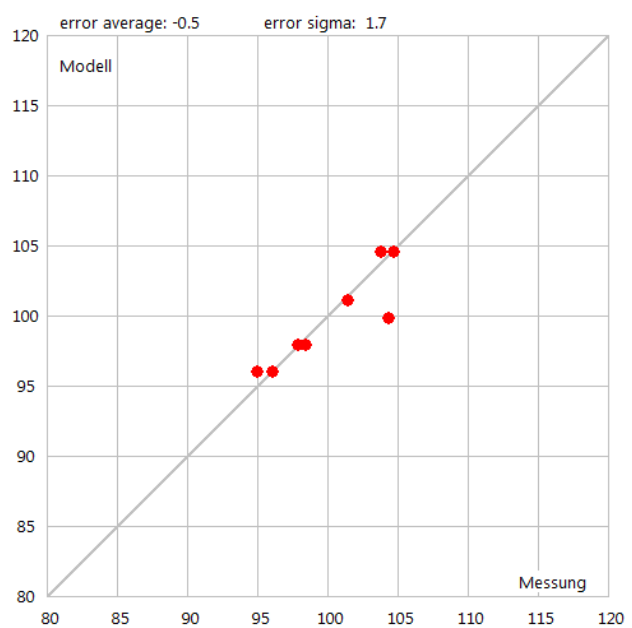
Abbildung 2: X-Y Plot der gemessenen und modellierten A-Summenpegel.
