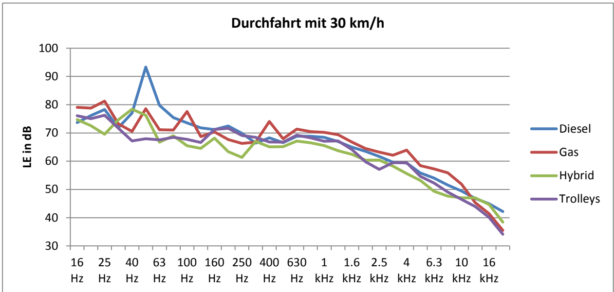
Abb. 6: Frequenzspektrum nach Antriebsart bei 30 km/h (ohne Belagsberücksichtigung)
