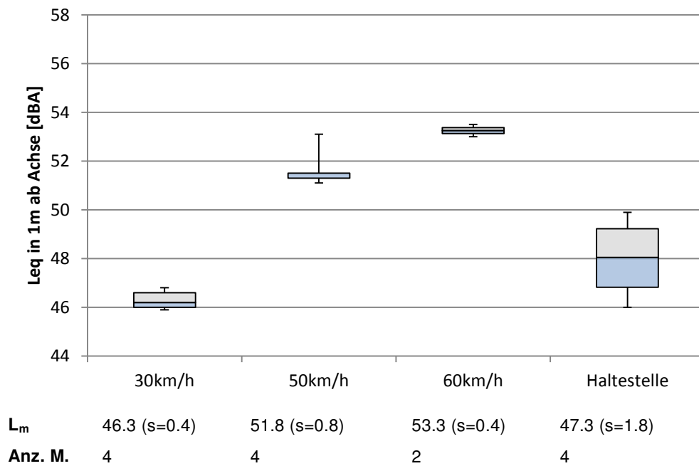
Abb. 18: Boxplots Kategorie Hybrid
