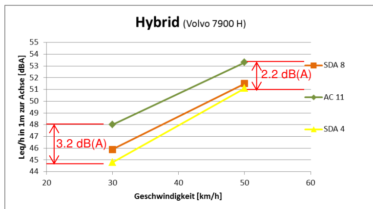
Abb. 11: Quellenwert (L q ) Hybrid
