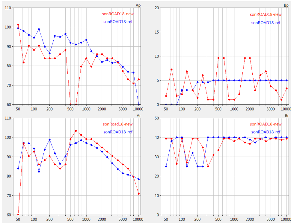
Abbildung 37: Spektrale Modellparameter in rot im Vergleich zu den Standardwerten SWISS10 cat 1 (blau).
