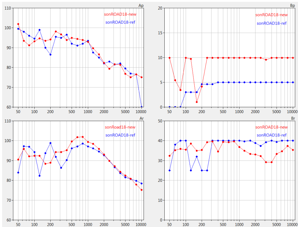
Abbildung 58: Spektrale Modellparameter in rot im Vergleich zu den Standardwerten SWISS10 cat 1 (blau).
