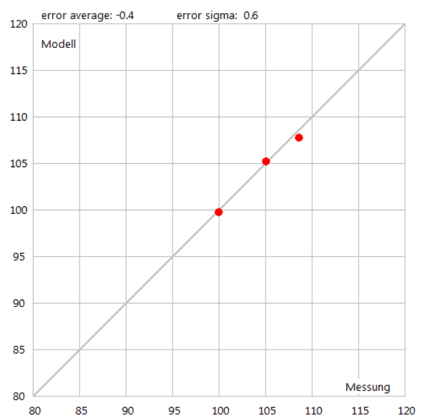
Abbildung 18: X-Y Plot der gemessenen und modellierten A-Summenpegel.
