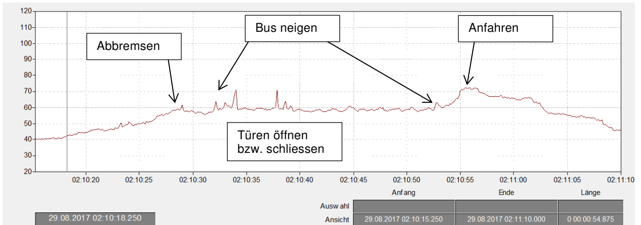
Abb. 25: Haltevorgang des Basler Bus Nr. 2, Gelenkbus, Kategorie Gas
