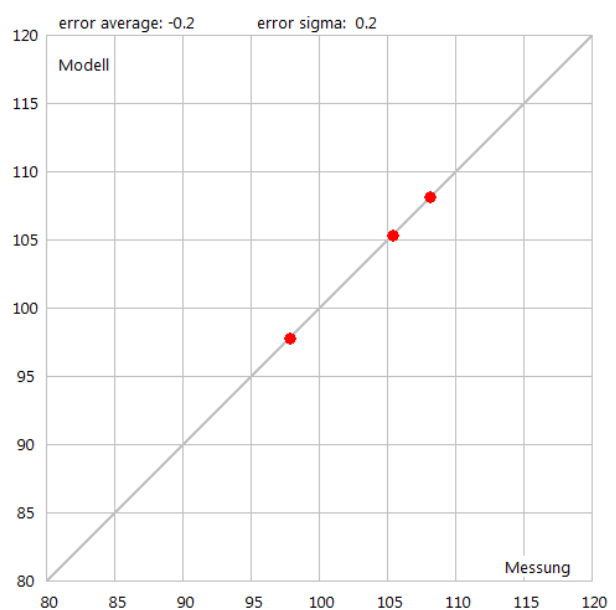
Abbildung 24: X-Y Plot der gemessenen und modellierten A-Summenpegel.
