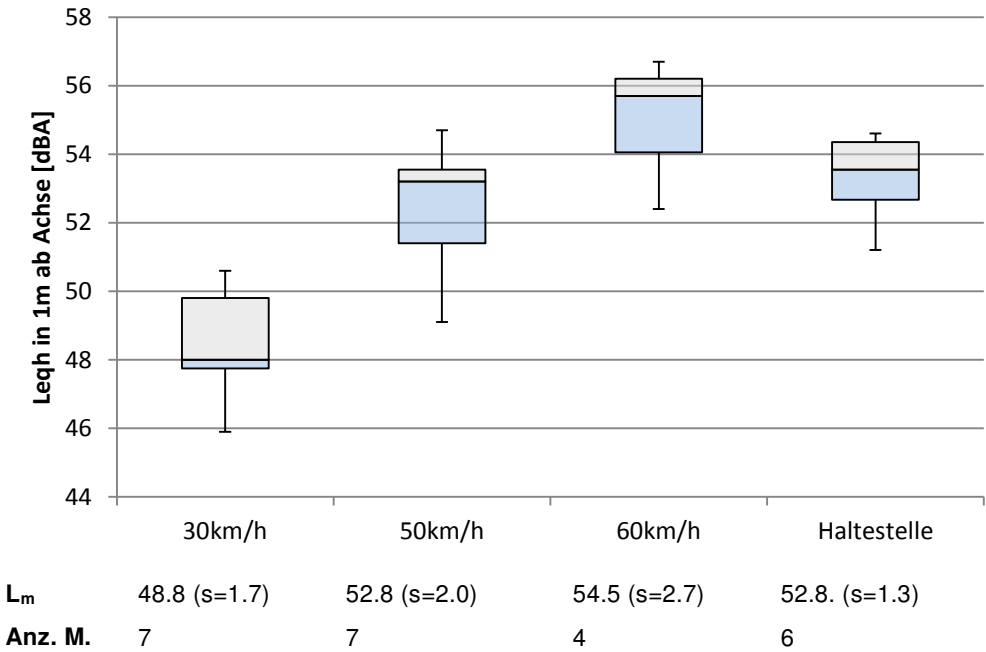
Abb. 15: Boxplots Kategorie Diesel, 2-Achser, Standardbus
