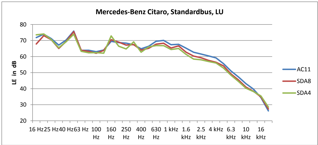
Abb. 2: Frequenzspektren unterschiedlicher Beläge des Luzerner Standardbusses mit Dieselantrieb, Schalldruckpegel in dB
