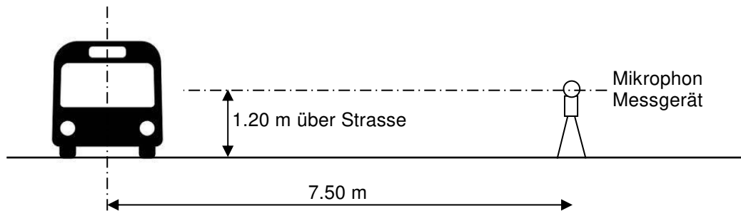
Abb. 1: Allgemeine Messanordnung
