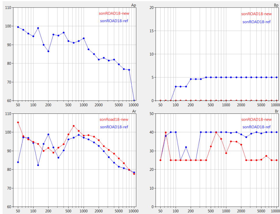
Abbildung 35: Spektrale Modellparameter in rot im Vergleich zu den Standardwerten SWISS10 cat 1 (blau).
