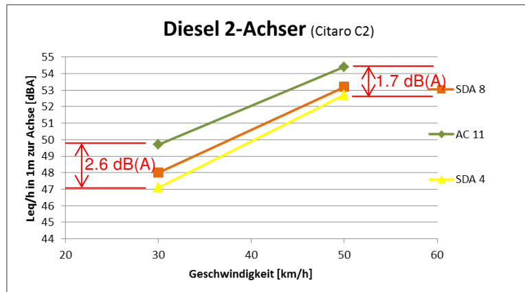
Abb. 10: Quellenwert (L q ) Diesel 2-Achser
