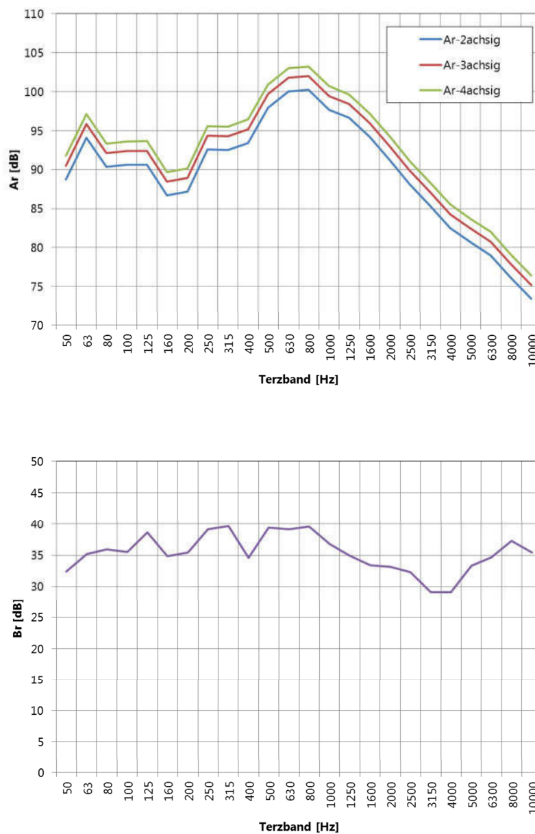
Abbildung 49: Mittlere achszahlabhängige Ar Spektren (oben) und mittleres Br Spektrum (unten).
