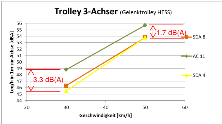
Abb. 12: Quellenwert (L q ) Trolley 3-Achser
