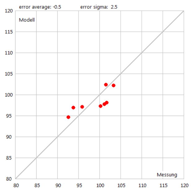
Abbildung 8: X-Y Plot der gemessenen und modellierten A-Summenpegel.
