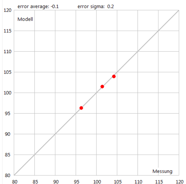
Abbildung 22: X-Y Plot der gemessenen und modellierten A-Summenpegel.
