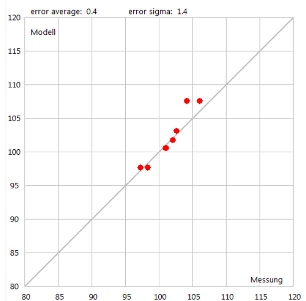
Abbildung 55: X-Y Plot der gemessenen und modellierten A-Summenpegel.
