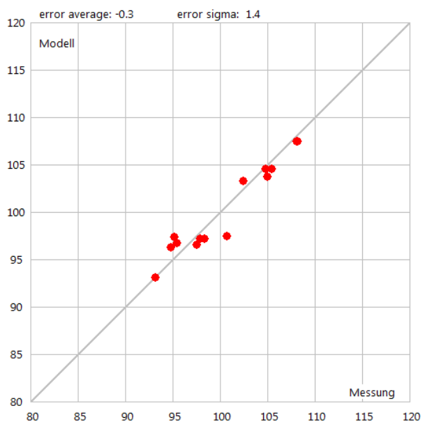
Abbildung 48: X-Y Plot der gemessenen und modellierten A-Summenpegel.
