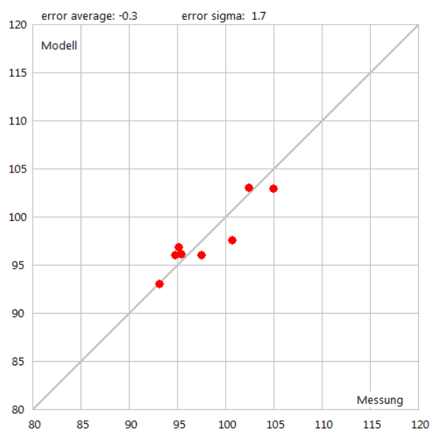
Abbildung 12: X-Y Plot der gemessenen und modellierten A-Summenpegel.
