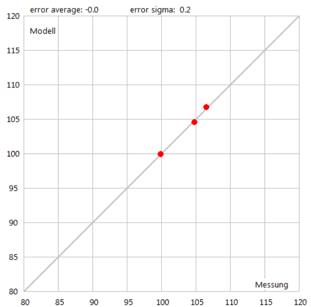
Abbildung 14: X-Y Plot der gemessenen und modellierten A-Summenpegel.
