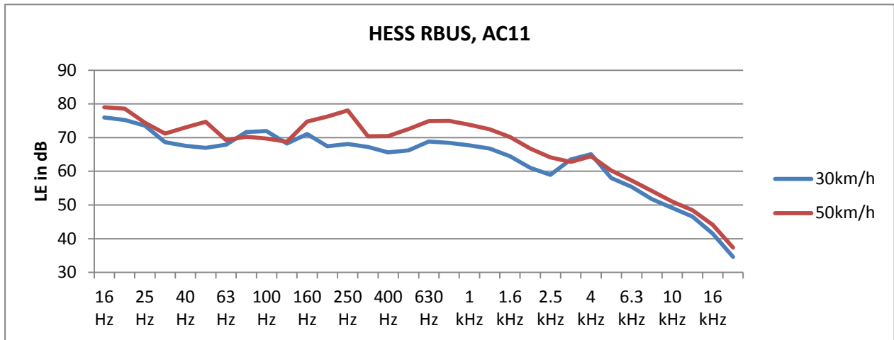
Abb. 8: Frequenzspektrum des Luzerner HESS RBUS
