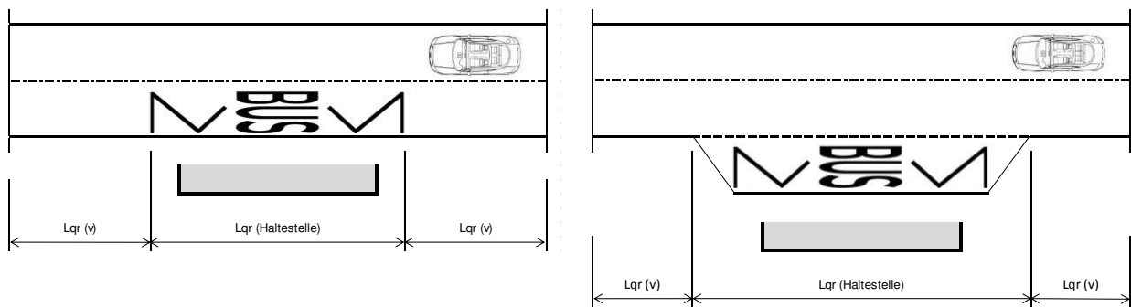
Abb. 27: Emissionsangaben im Bereich von Haltestellen
