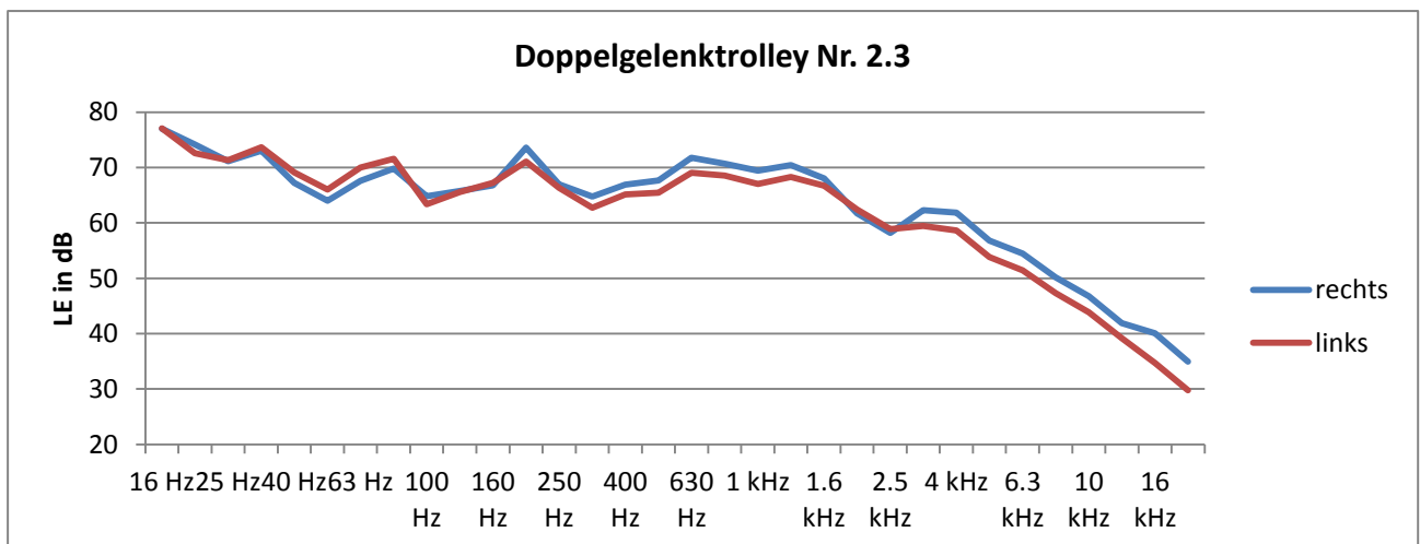
Abb. 3: Frequenzspektren links und rechts des Züricher Doppelgelenktrolleys Nr. 2.3, Schalldruckpegel in dB
