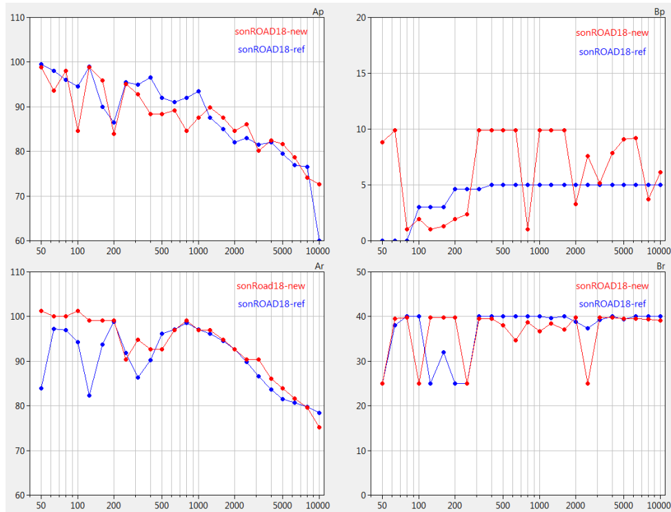
Abbildung 21: Spektrale Modellparameter in rot im Vergleich zu den Standardwerten SWISS10 cat 1 (blau).
