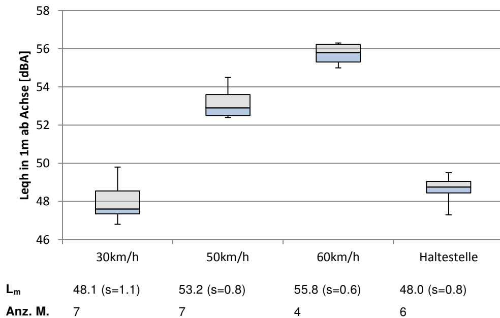
Abb. 20: Boxplots Kategorie Trolley, 4-Achser, Doppelgelenktrolleybus
