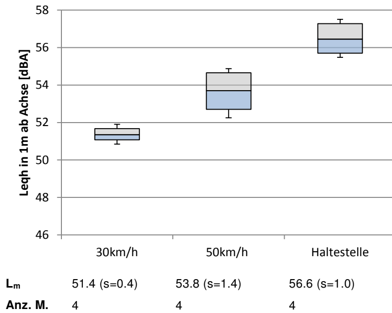
Abb. 17: Boxplots Kategorie Gasbus
