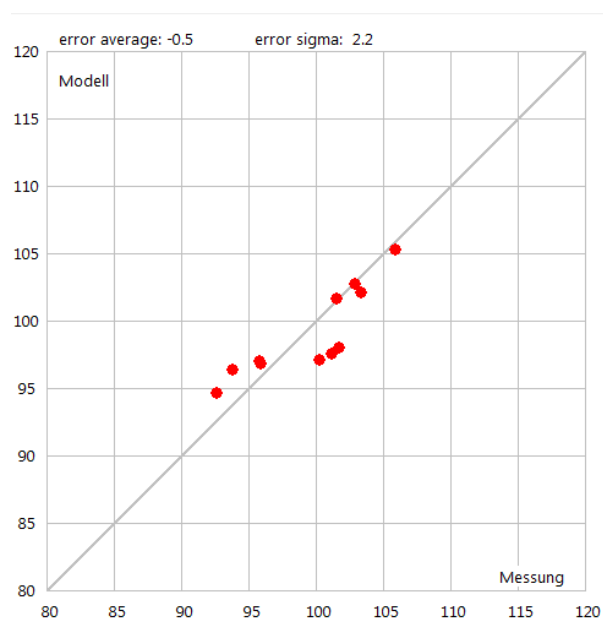
Abbildung 44: X-Y Plot der gemessenen und modellierten A-Summenpegel.
