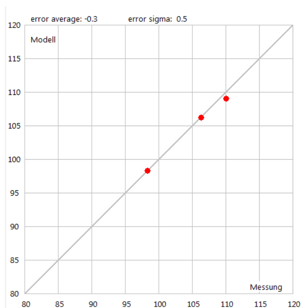
Abbildung 28: X-Y Plot der gemessenen und modellierten A-Summenpegel.
