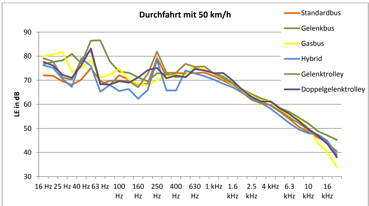
Abb. 5: Frequenzspektren der verschiedenen Kategorien bei einer Durchfahrt mit 50 km/h (ohne Belagsberücksichtigung)
