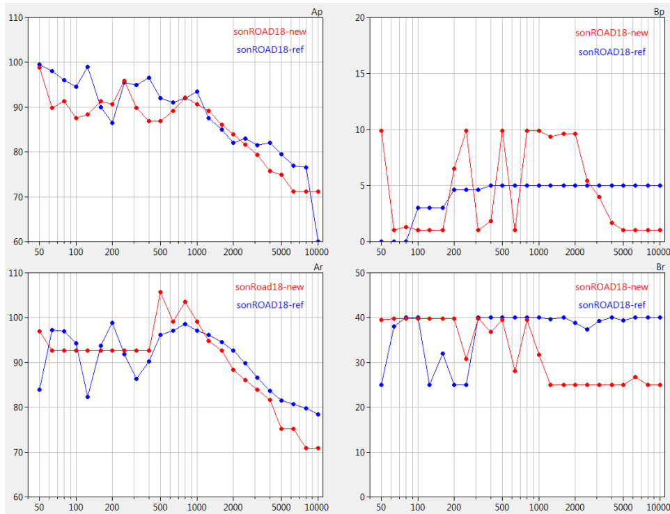
Abbildung 7: Spektrale Modellparameter in rot im Vergleich zu den Standardwerten SWISS10 cat 1 (blau).
