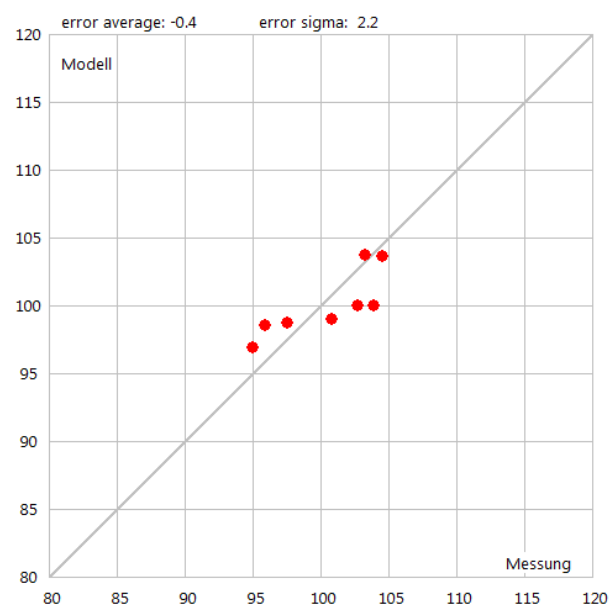
Abbildung 6: X-Y Plot der gemessenen und modellierten A-Summenpegel.
