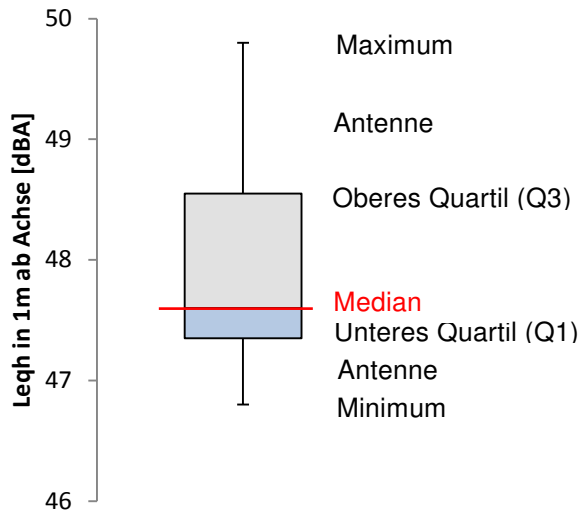
Abb. 14: Definitionen Boxplot
