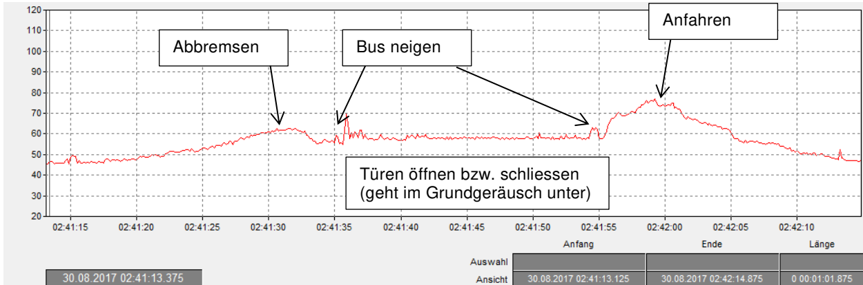
Abb. 24: Haltevorgang des Basler Gelenkbus, Kategorie Diesel
