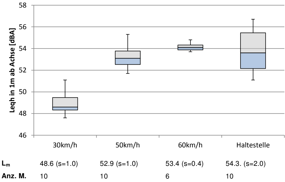
Abb. 16: Boxplots Kategorie Diesel, 3-Achser, Gelenkbus
